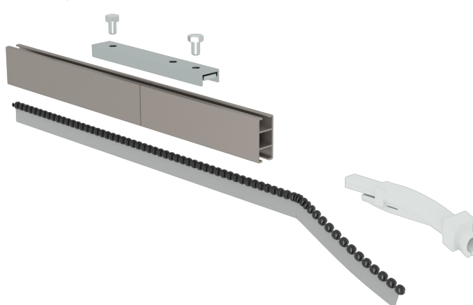
RapidSlider
