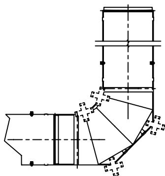
Codos de 2 pliegues ( < 70^\circ ) con correas de longitud estándar
