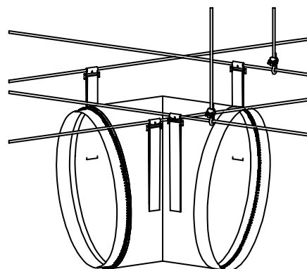
Codos de 4 pliegues ( \geq 70^\circ ) con correas extendidas.
