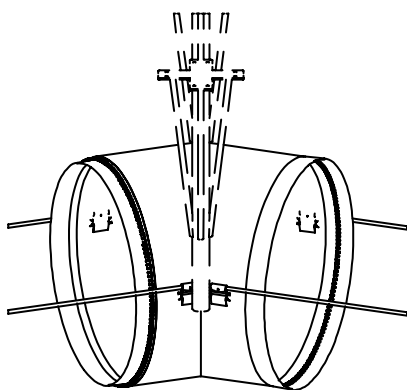
Codos de 4 pliegues ( \geq 70^\circ ) con correas de longitud estándar.
