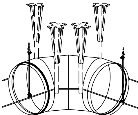
Codos de 4 pliegues ( \geq 70^\circ ) con correas de longitud estándar.
