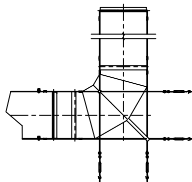
Codos de 2 pliegues ( < 70^\circ ) con correas de longitud estándar.
