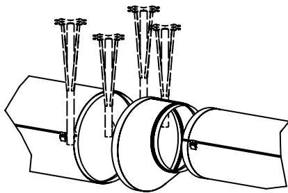
Reducciones Alineadas en la parte superior/ centro/inferior
