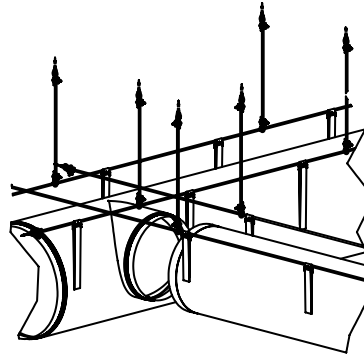
Ramificaciones Alineadas en la parte superior/ centro/inferior
