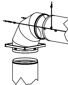
Métodos de suspensión de conductos verticales
