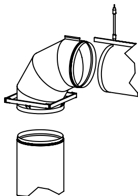
Métodos de suspensión de conductos verticales
