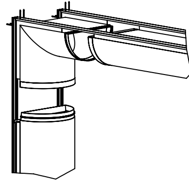
Dikey askı sistemi montaj seçenekleri
